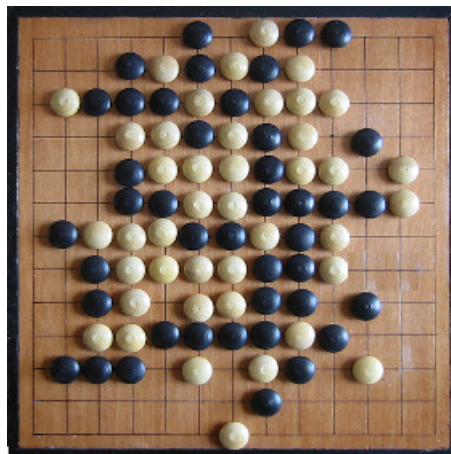
Figura 5.2: Desafio Gomoku
